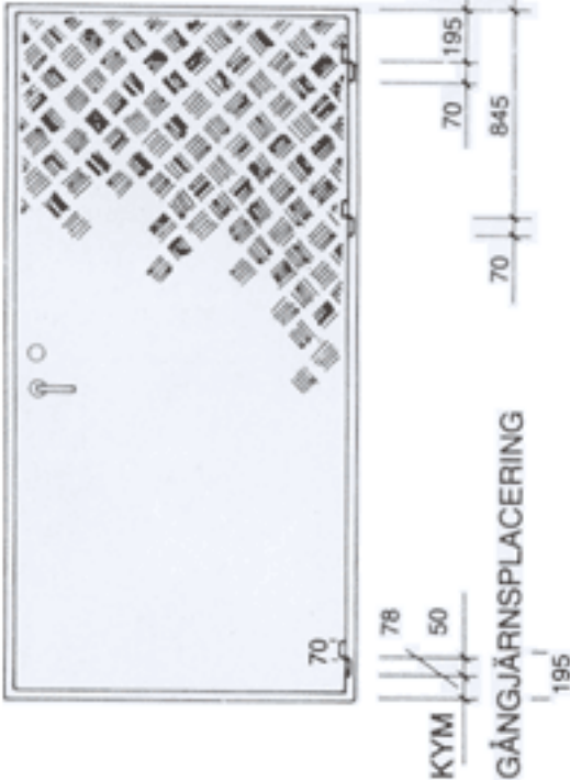
Enkeldörr med isolerruta
