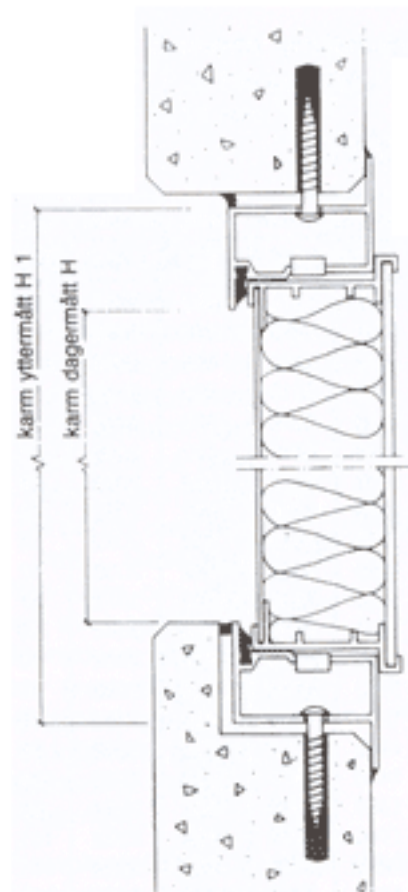
Vertikalsektion
